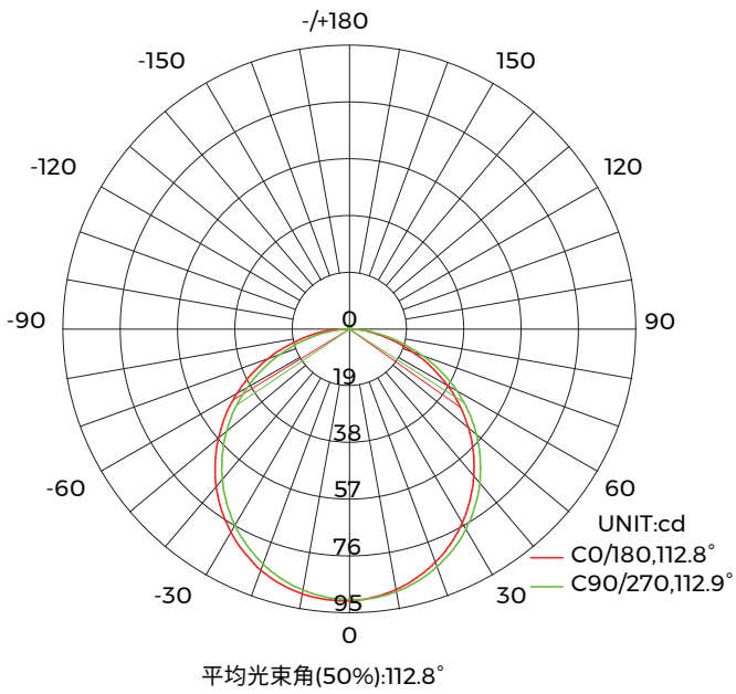
配光曲线
