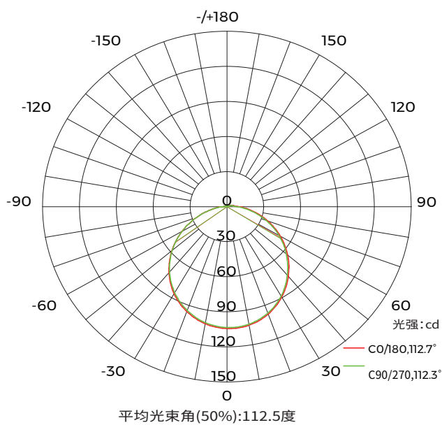
配光曲线
