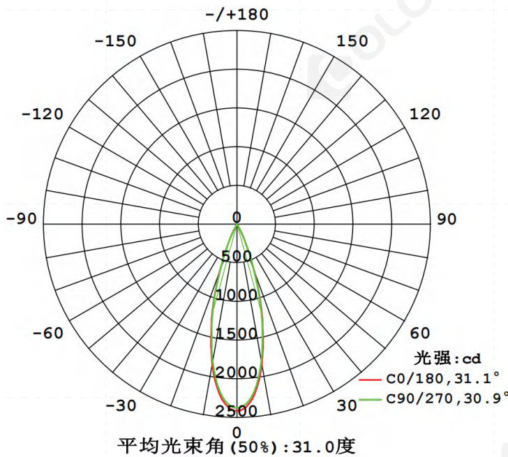
配光曲线图
