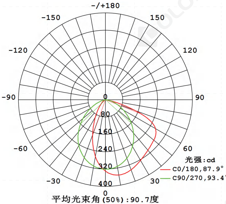
配光曲线图
