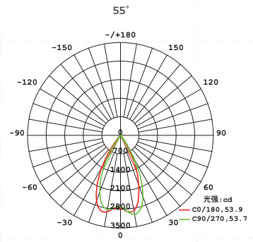
平均光束角(50%):53.8度
