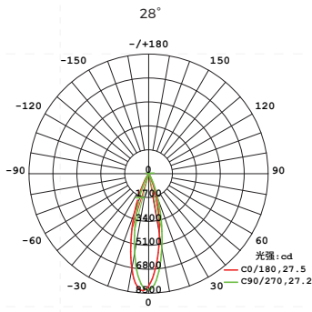
平均光束角(50%):27.4度
