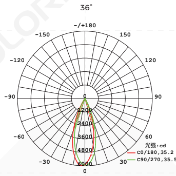
平均光束角(50%):35.4度
