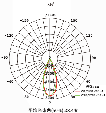
配光曲线
