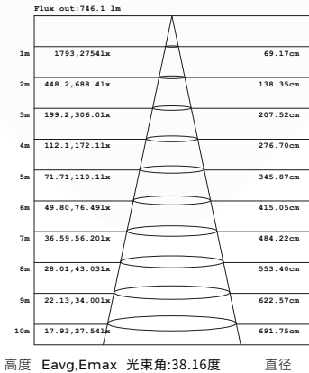
配光曲线
