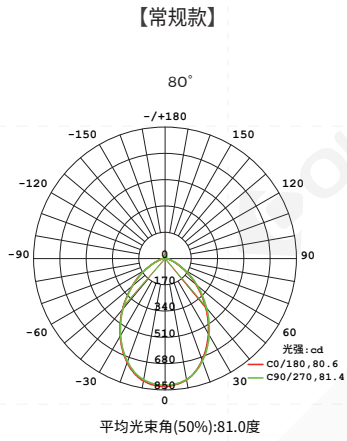
配光曲线
