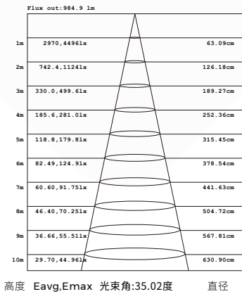
配光曲线
